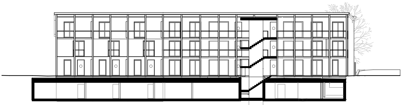
Ansicht Ost, Haus D
